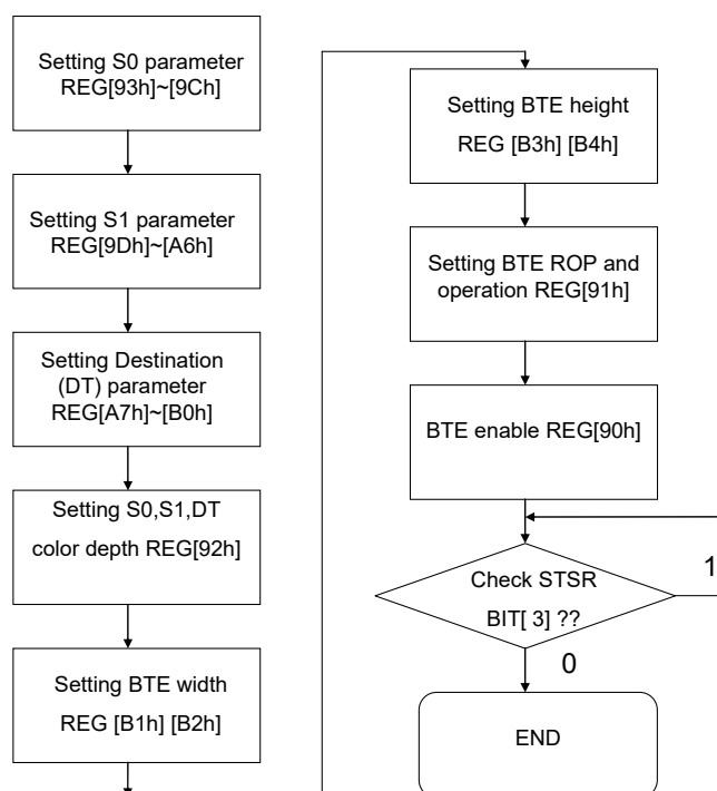
圖 4-28：流程图
