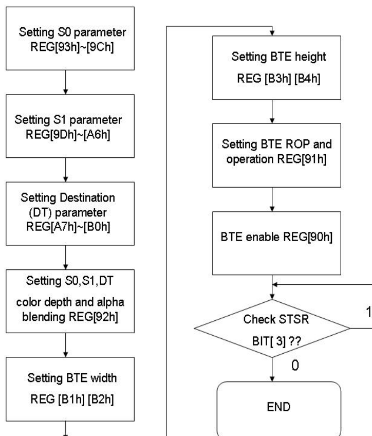
圖 4-6 : 流程图
