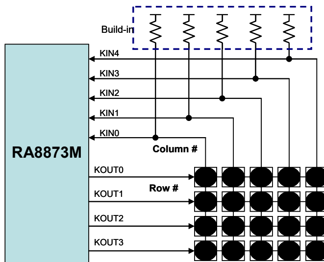
圖 8-3：Key-Pad Application
