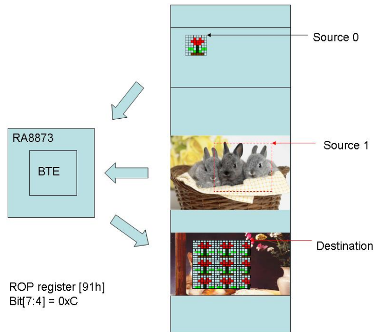
圖 4-72：硬件数据流
