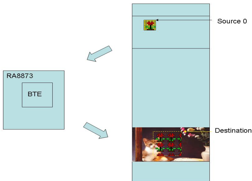
圖 4-10：硬件数据流
